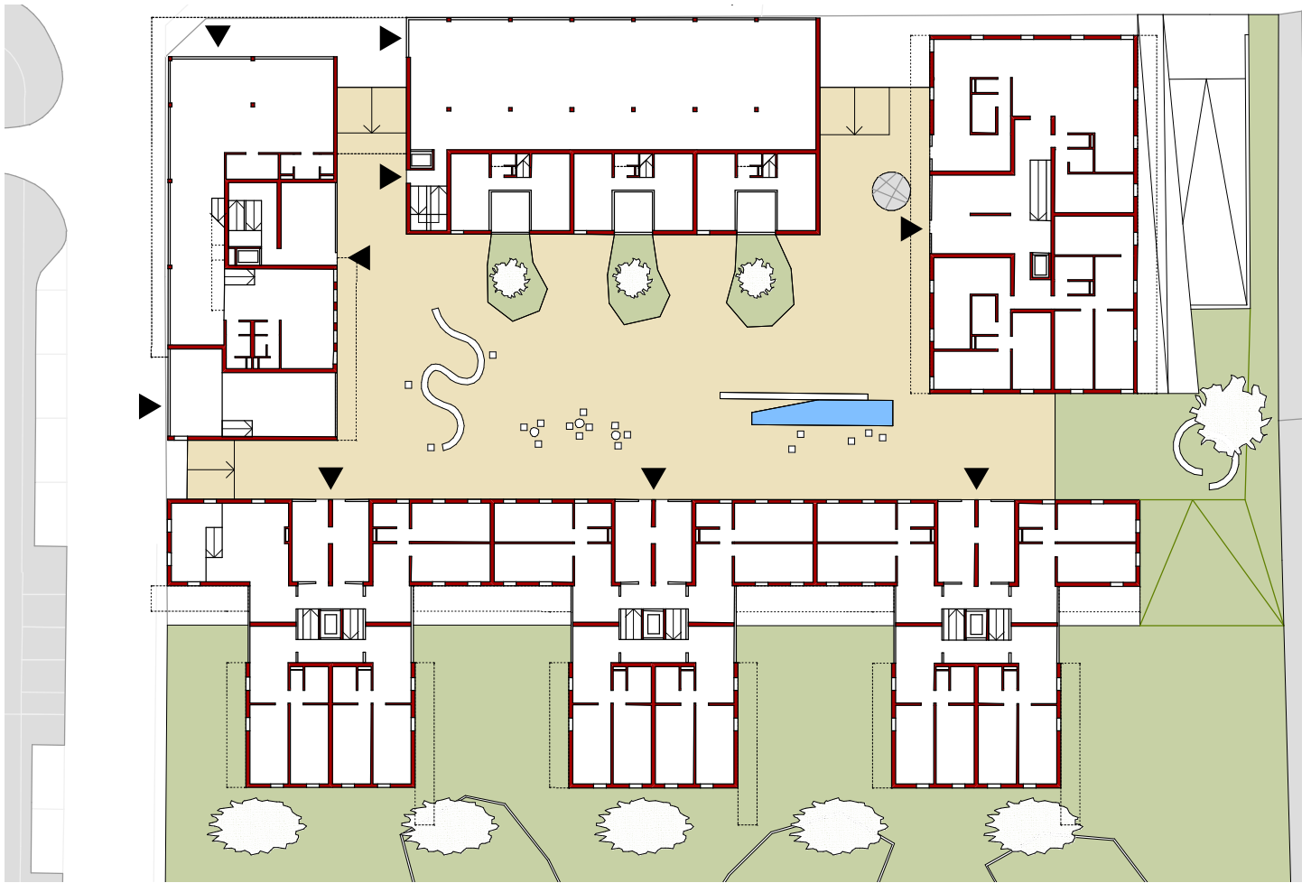
Erdgeschoss
