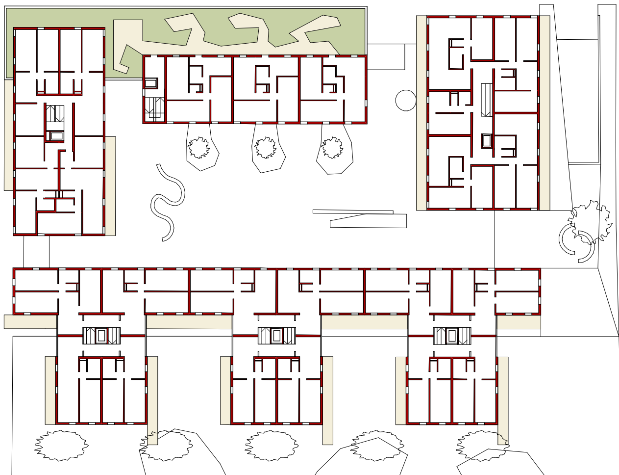
2. Obergeschoss
