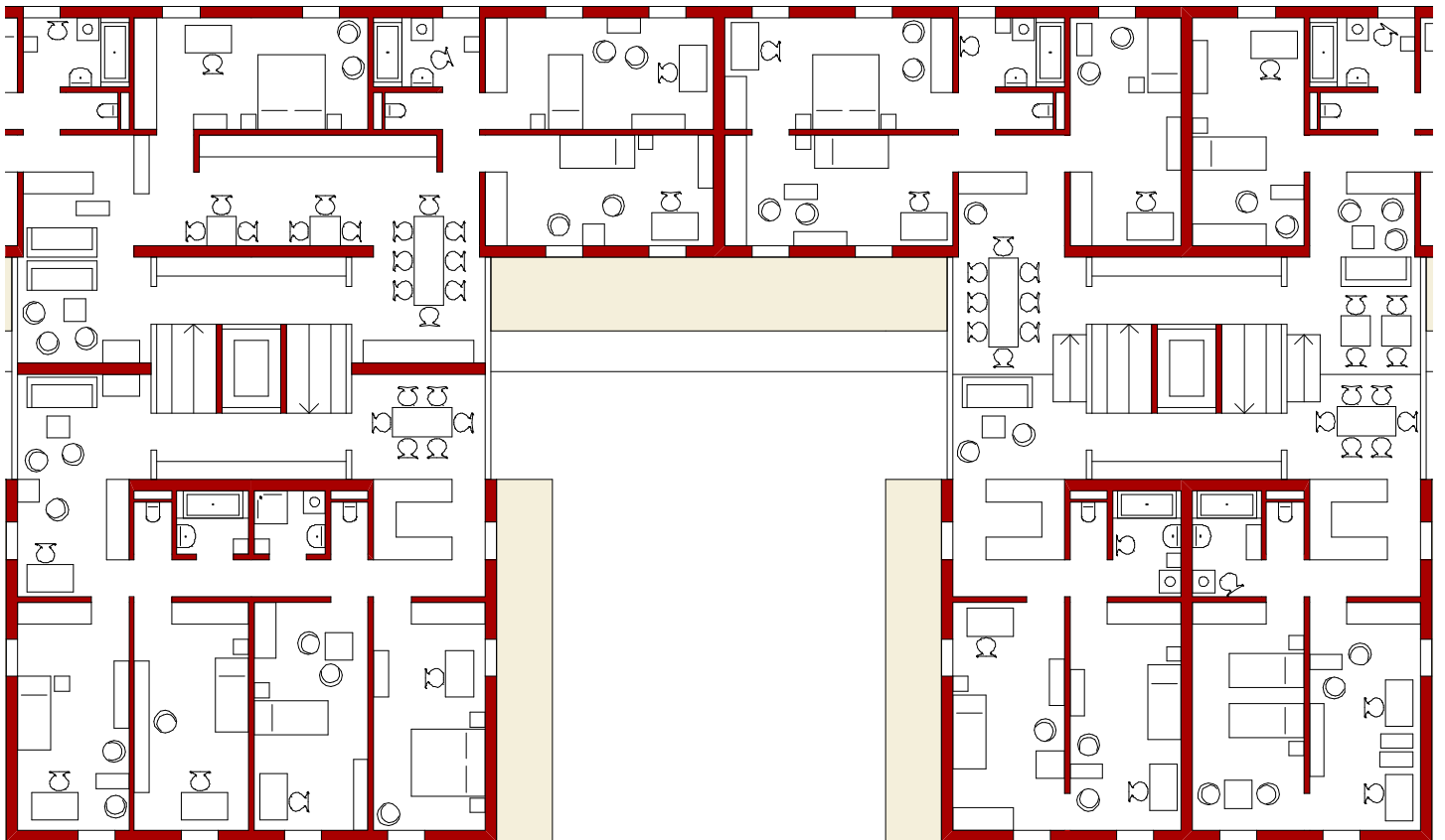
variable Wohnungsgrundrisse
